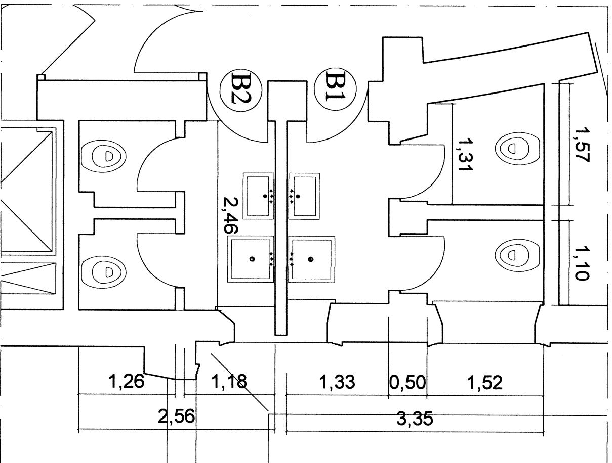
Planimetria bagni al terzo piano - Scala 1:50
